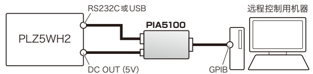
【连接示例】
