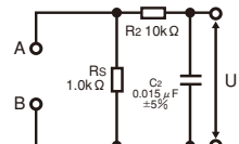
● 测量回路网(网络I IEC60601-1等)
