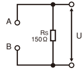
● 测量回路网(网络PCC-2 IEC60598-1)
