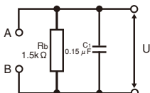
● 测量回路网(网络F IEC61029等)
