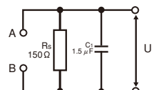
● 测量回路网(网络PCC-2 IEC60598-1)
